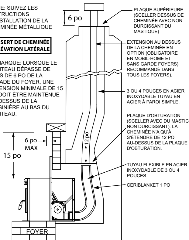
INSTALLATION DE TUYAU D'ÉCHAPPEMENT
